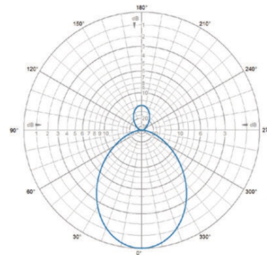
E-Plane | 445 MHz
