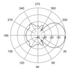
E-Plane | 165 MHz
