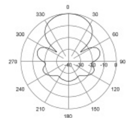
H-Plane | 165 MHz
