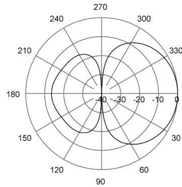
E-Plane | 153 MHz
