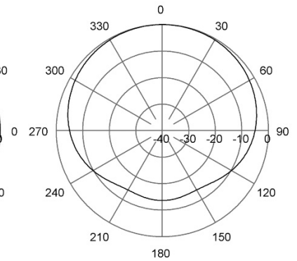
H-Plane | 153 MHz
