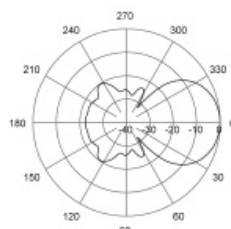
E-Plane | 155 MHz
