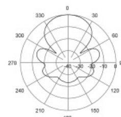
H-Plane | 155 MHz
