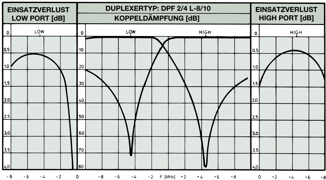
TYPISCHER KURVENVERLAUF @ 9 MHz DUPLEXABSTAND:
