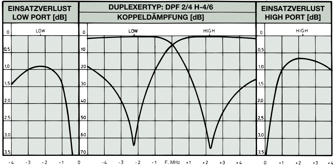
TYPISCHER KURVENVERLAUF @ 4.5 MHz DUPLEXABSTAND:
