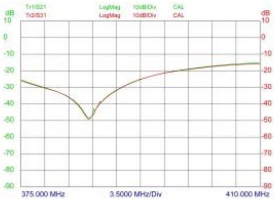
TYPISCHER KURVENVERLAUF ANTENNEN MU 3-BZ/TETRA/L (MIT 1.5 M KABEL)
