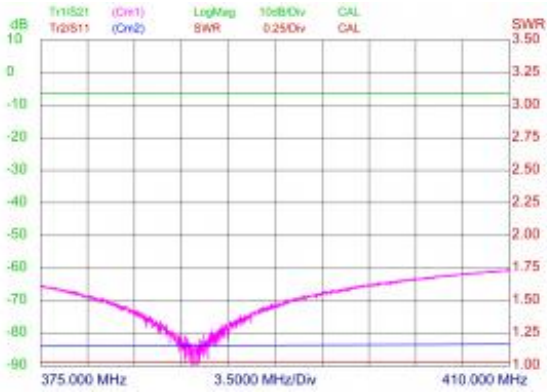
TYPISCHER KURVENVERLAUF SWR 1
