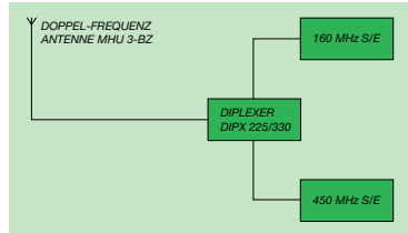
KOPPELDIAGRAMM:
