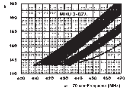
2 m-Frequenz (MHz)
