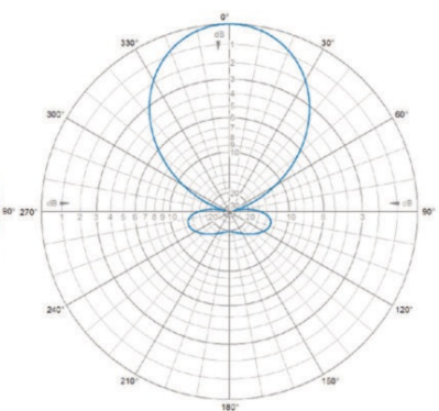
H-Plane | 405 MHz
